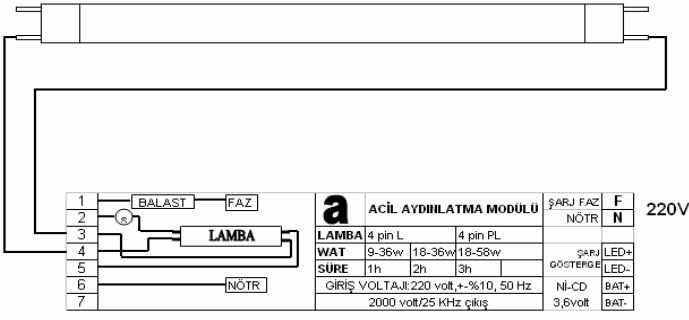
Düz Çubuk Floresan Acilde Yanan Bağlantısı
