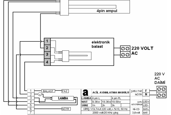
Elektronik Balastlı 4 Pin PL Ampul Sürekli Bağlantısı
