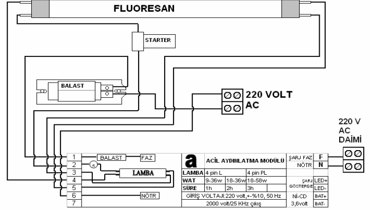
Düz Çubuk Floresan Sürekli Yanan Bağlantısı
