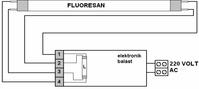
Elektronik Balastlı Düz Çubuk Ampul Şebeke Bağlantısı
