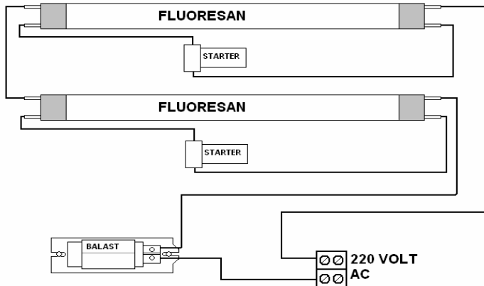
1 Magnetik Balastlı, 2 düz fluoresent lambalı Şebekeden yanar bağlantı
