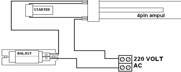
Düz Çubuk Floresan Şebekeden Yanan Bağlantısı
