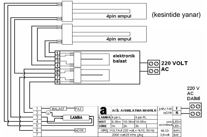
Elektronik Balastlı 2 Adet 4 Pin PL Sürekli Bağlantısı 1 Lamba Acilde Yanar
