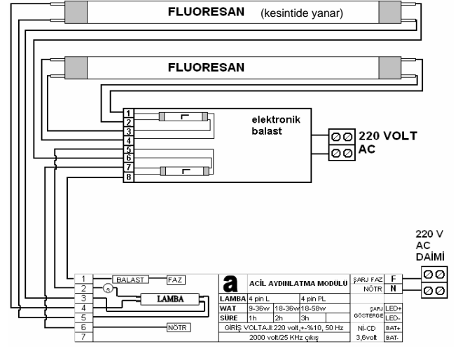
Elektronik Balastlı 2 Fluoresan Sürekli Bağlantısı 1 Lamba acilde yanar
