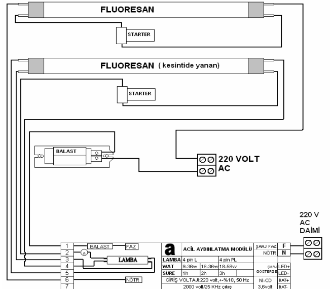
1 Magnetik Balastlı, 2 lamba, sürekli yanar bağlantısı Şebekeden 2 lamba, kesintide 1 lamba yanar
