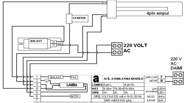
4 Pin PL Floresan Sürekli Yanan Bağlantısı
