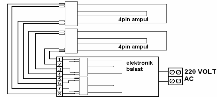
Elektronik Balastlı 2 Adet 4 Pin PL Şebeke Bağlantısı
