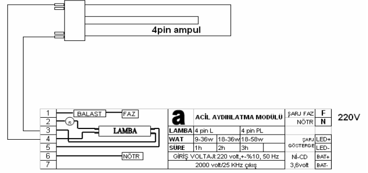
4 Pin PL Ampul Acilde Yanan Bağlantısı
