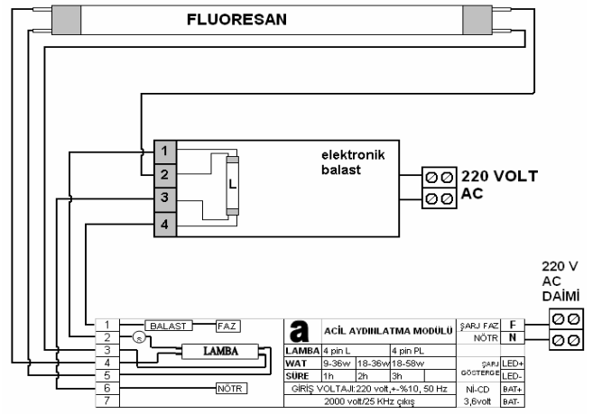
Elektronik Balastlı Düz Çubuk Ampul Sürekli Bağlantısı
