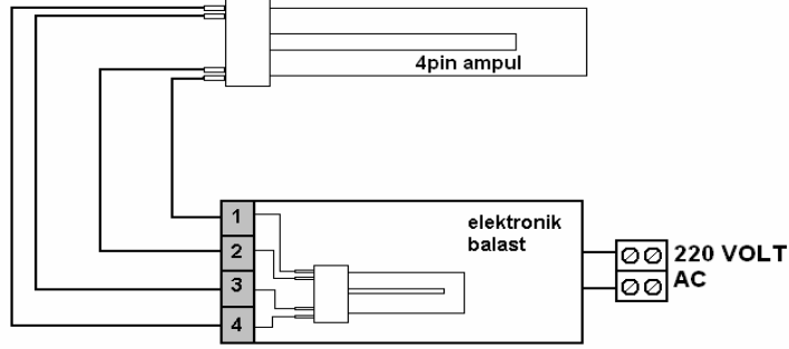
Elektronik Balastlı 4 Pin PL Ampul Şebeke Bağlantısı
